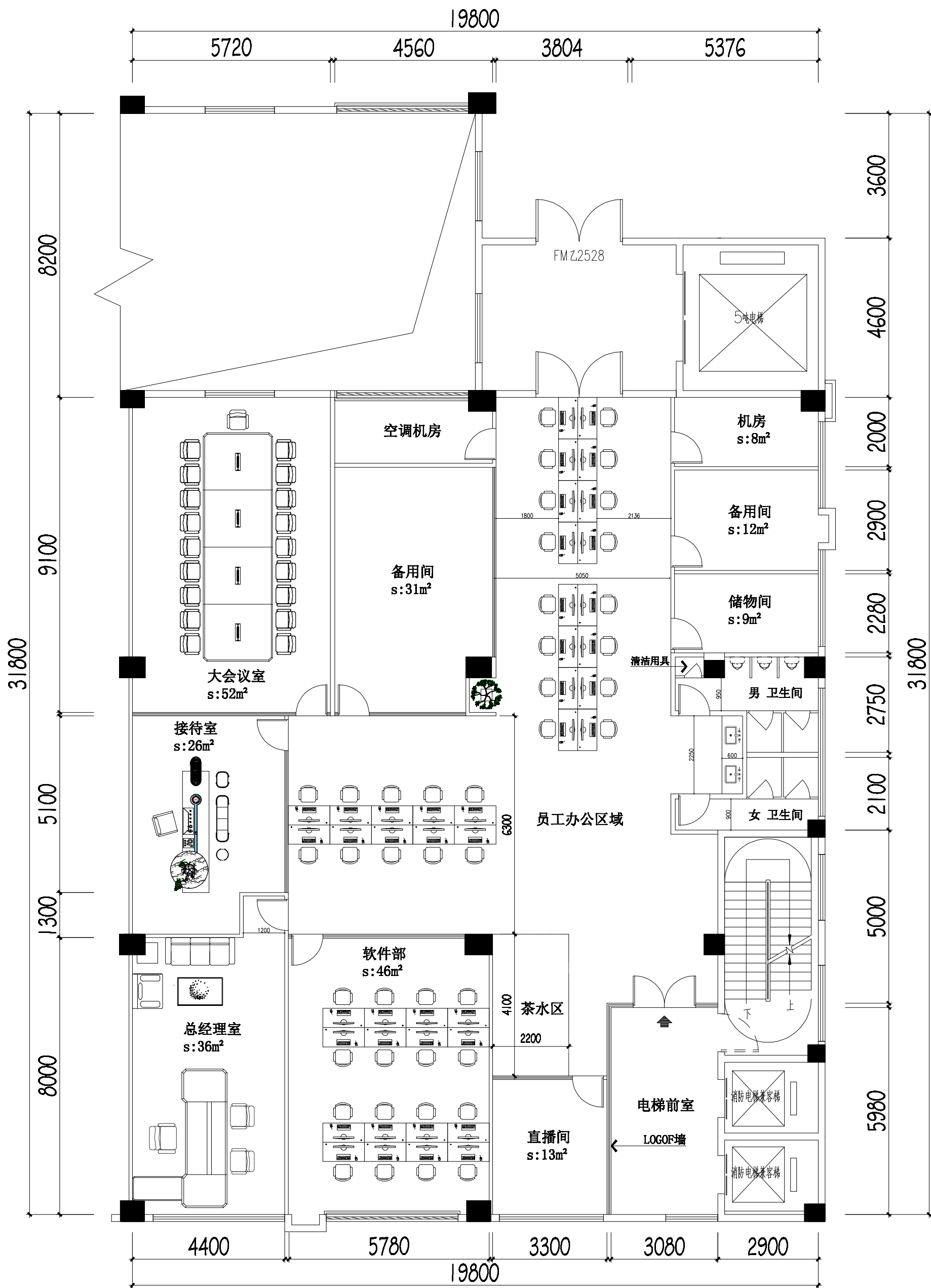
平面方案布置图
